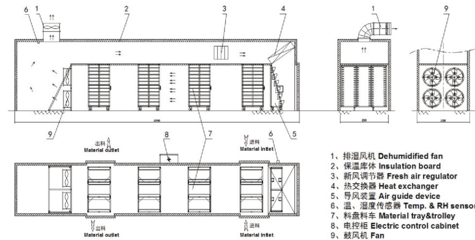
HGS型隧道式烘干机示意图 HGS tunnel dryer Sketch Map
