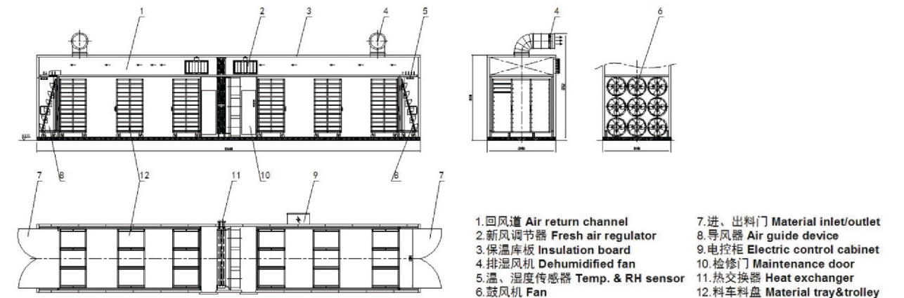
HGS-D型隧道式低温烘干机示意图 HGS-D low temperature tunnel dryer Sketch Map
